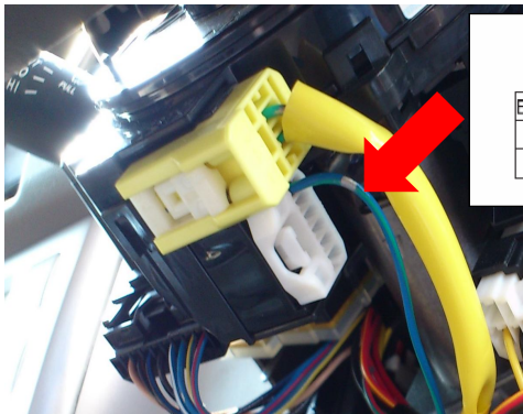
コネクタ3 センターパネル下を外すとコネクタが出てきます。2つコネクタがありますが、使用するのは下側です。
