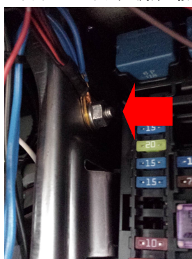
ポディーアース ヒューズボックス左のボディ金属部へ接続
