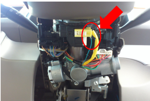
コネクタ2 運転席・コラムカバー下側を外した状態
