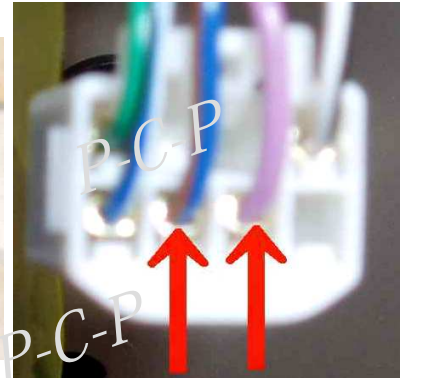
コネクタ2
